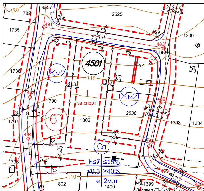
М 1:1000
