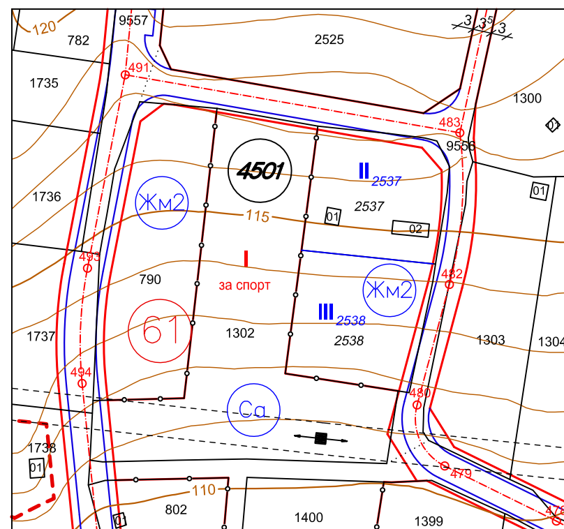
М 1:1000
