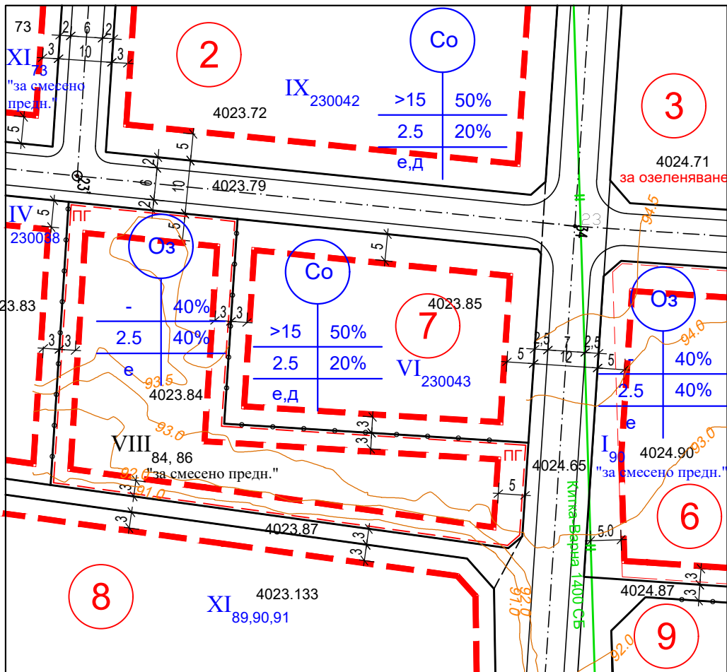
ПЛАН за ЗАСТРОЯВАНЕ М 1 : 1000
