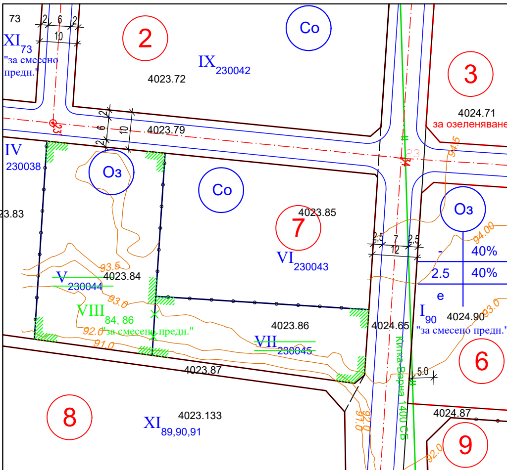
ПЛАН за РЕГУЛАЦИЯ М 1 : 1000
